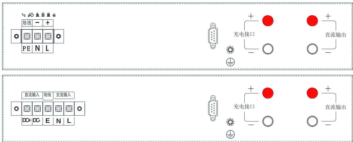
(图12-6) B 型机箱双路输入后面板
