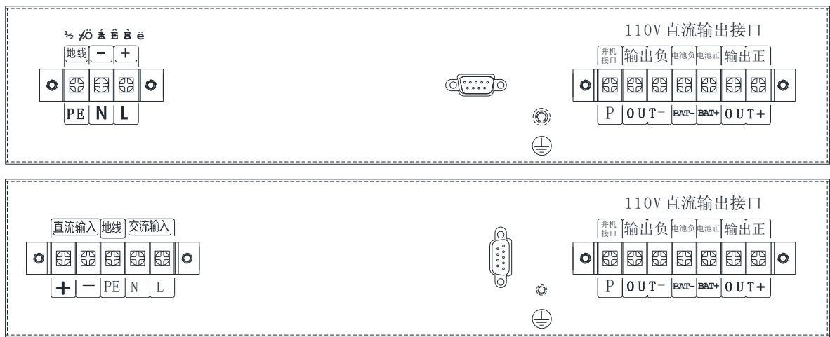
(图12-4) A 型机箱双路输入后面板
