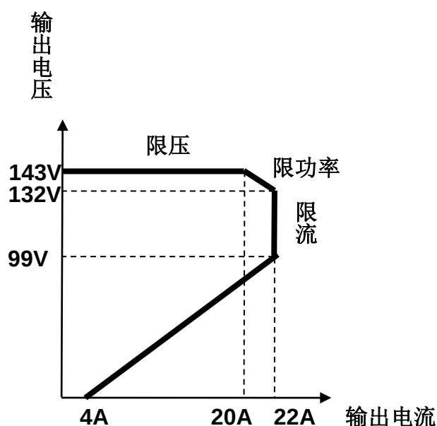
输出电流-输出电压转换曲线图（如下图所示）
