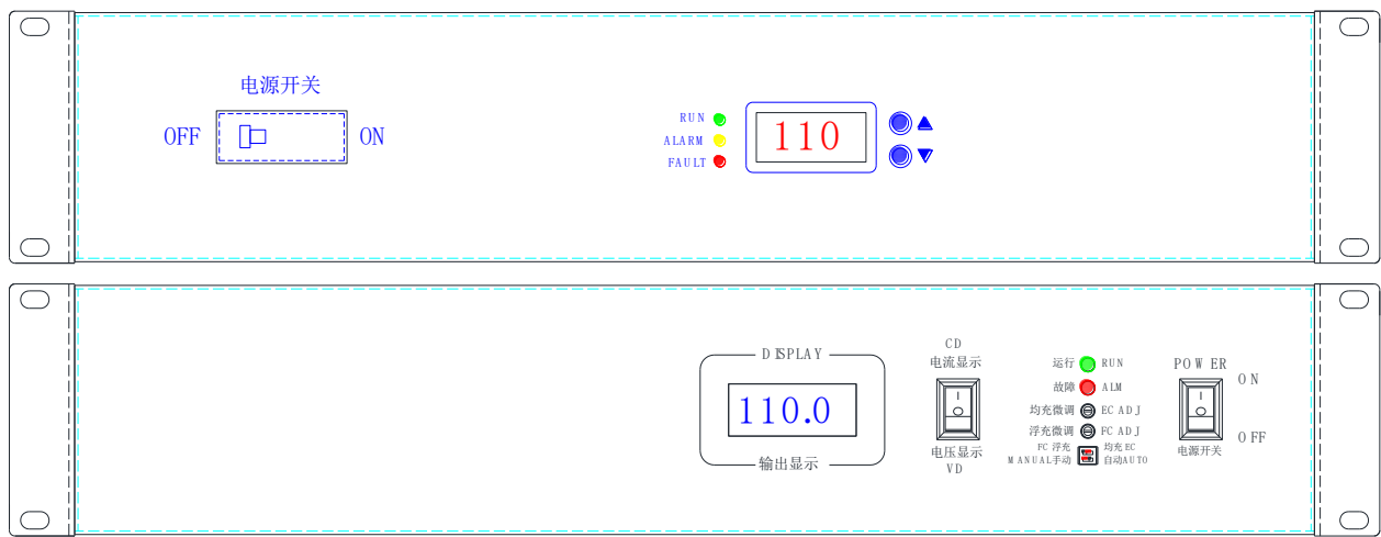
(图12-2) 表头型显示屏前面板图
