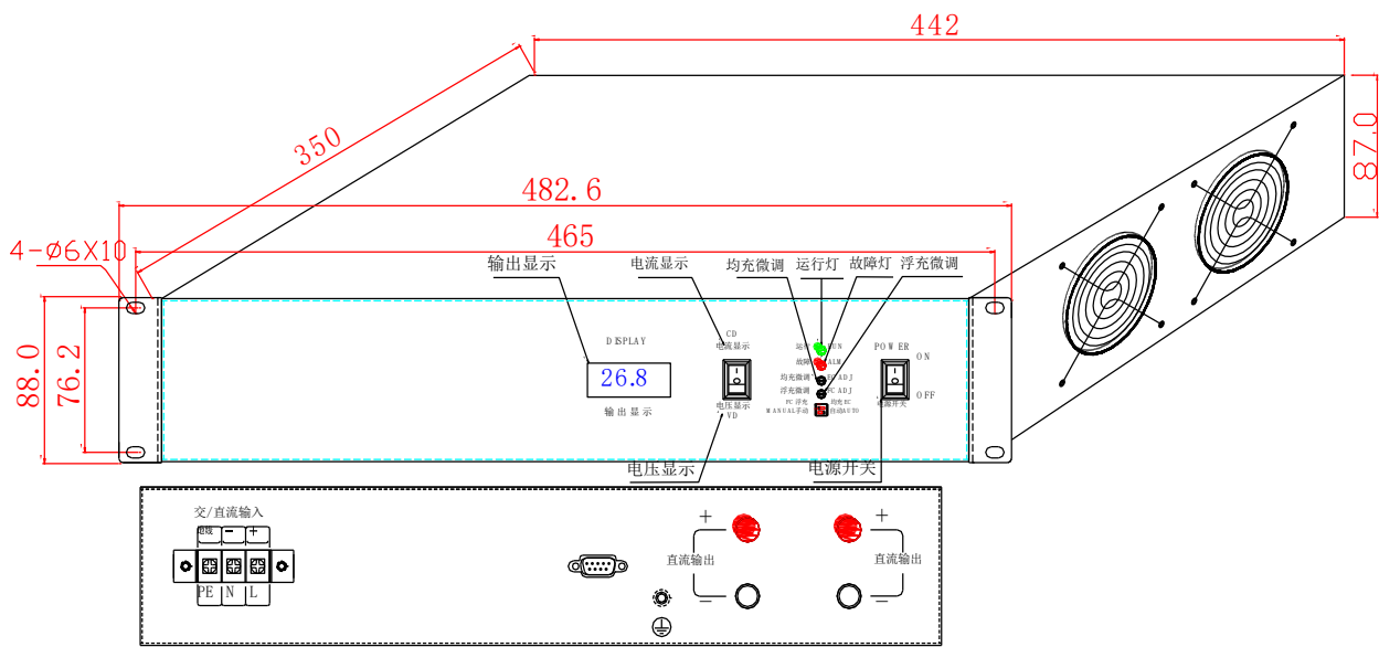
24100-2U机箱外形尺寸图
