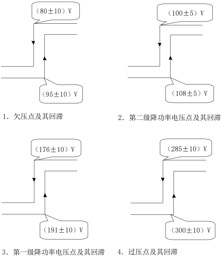
图4-1 交流输入过欠压保护点示意图
