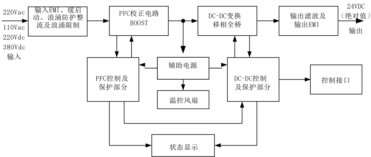
图2-4 24100-2U原理框图
