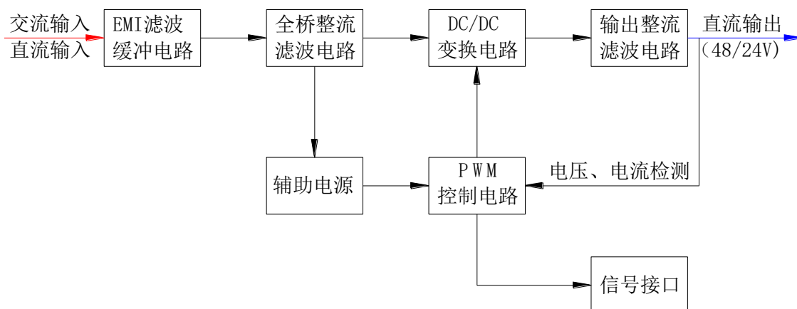
图 5-1 2430-2U 电源模块工作原理框图
