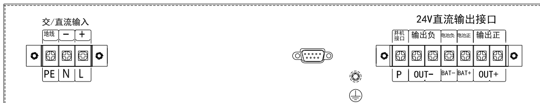
(图6) A型机箱后面板图
