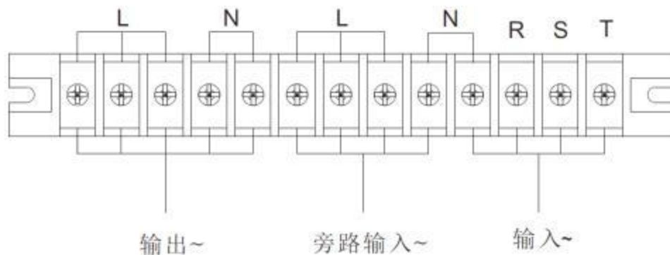
31 10K-20K 双输入端子台示意图
