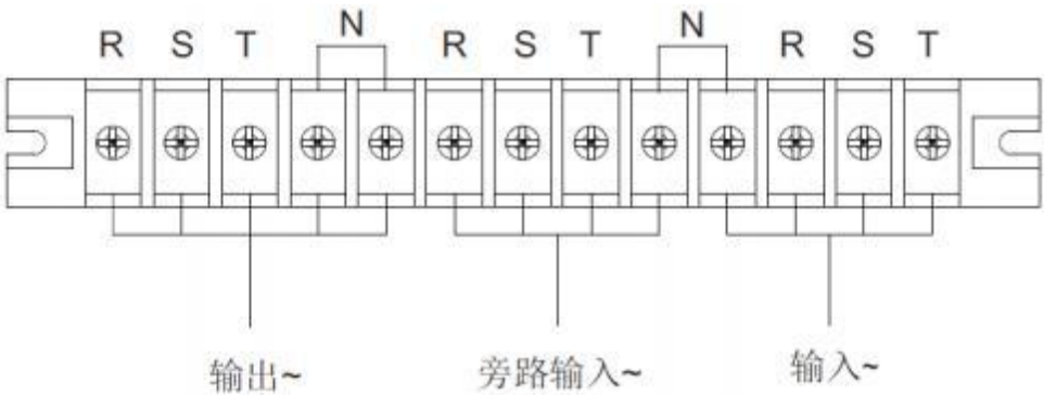
33 10K-30K 双输入端子台示意图
