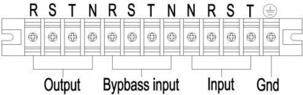
33 40K 双输入端子台示意图
