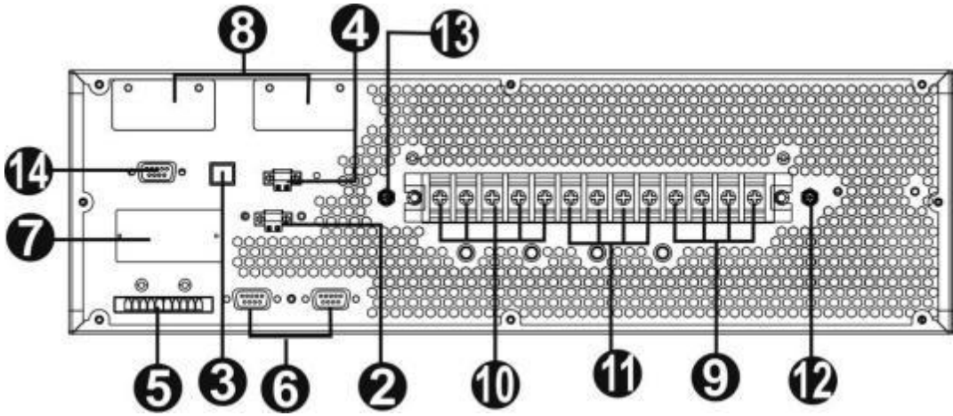
图 2: 后背板 输入/输出端子台
