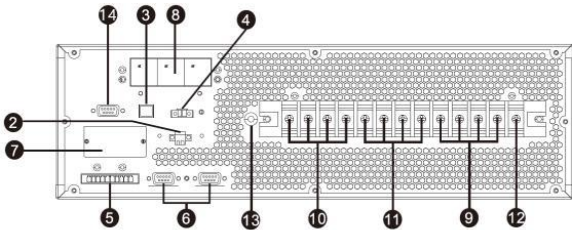
图 3：后背板 输入/输出端子台
