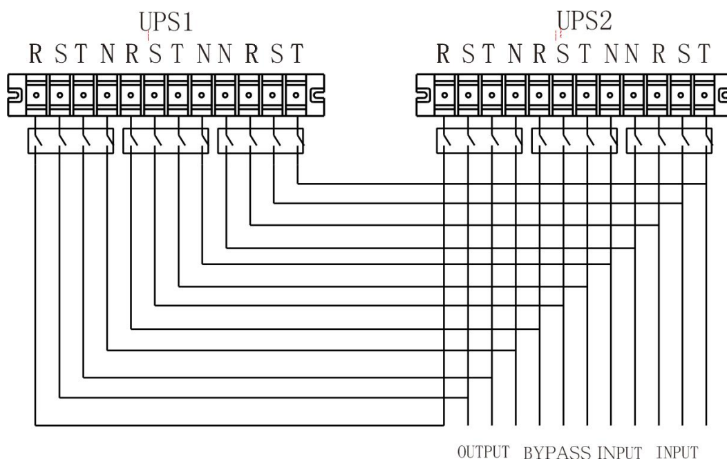
60K(S) 双输入并机系统接线图
