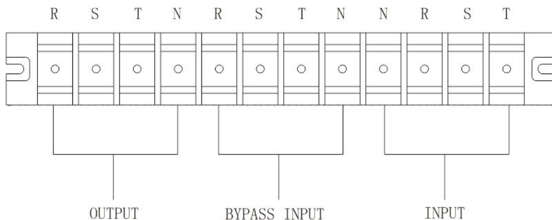
双输入 HV 60K(S)端子排示意图
