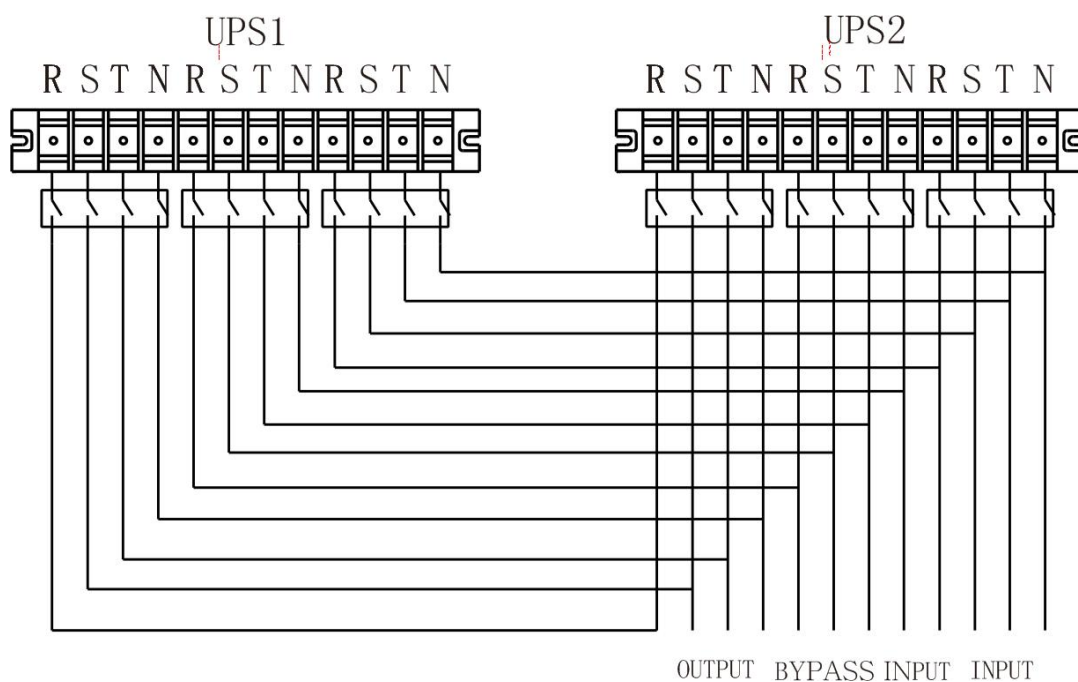
30K(S)/40K(S)双输入并机系统接线图
