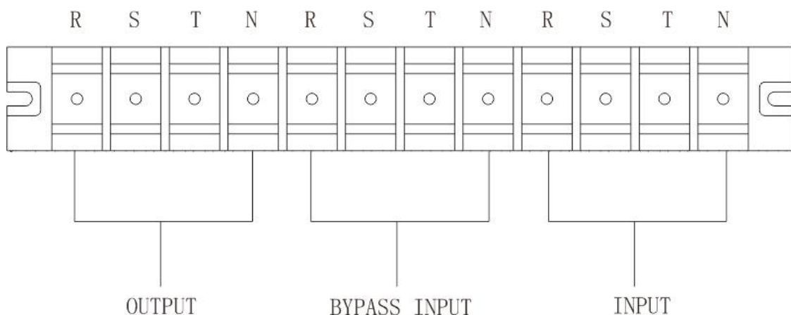
双输入 HV 30K(S)/40K(S) 端子排示意图
