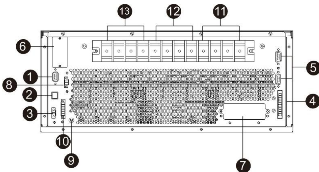
40K 后备板图
