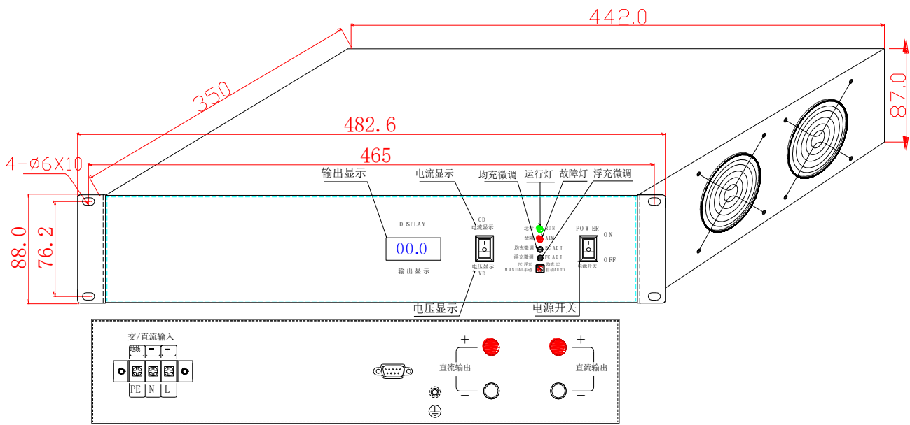
48100机箱外形尺寸图
