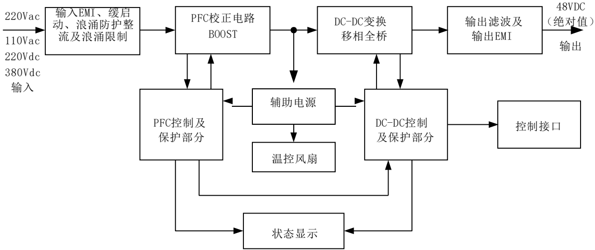
图2-4 48100-2U原理框图
