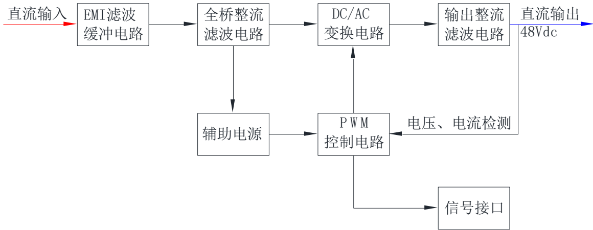
图 5-1 DC110-4830 直流变换电源工作原理框图
